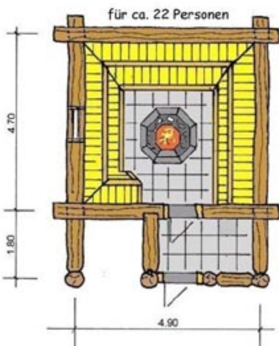
Grundriss
