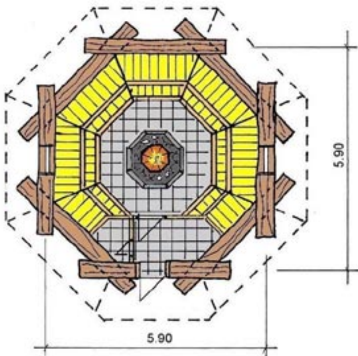
Grundriss
