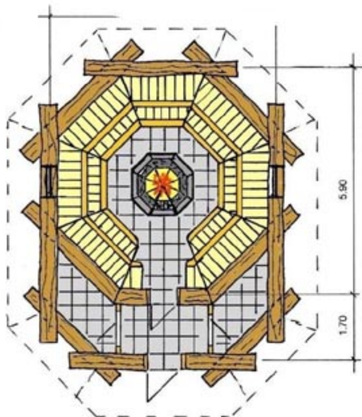
Grundriss
